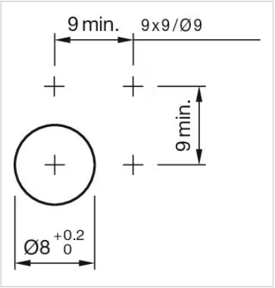
寸法図:
