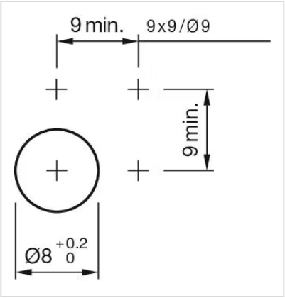
寸法図:
