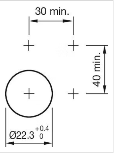
寸法図:
